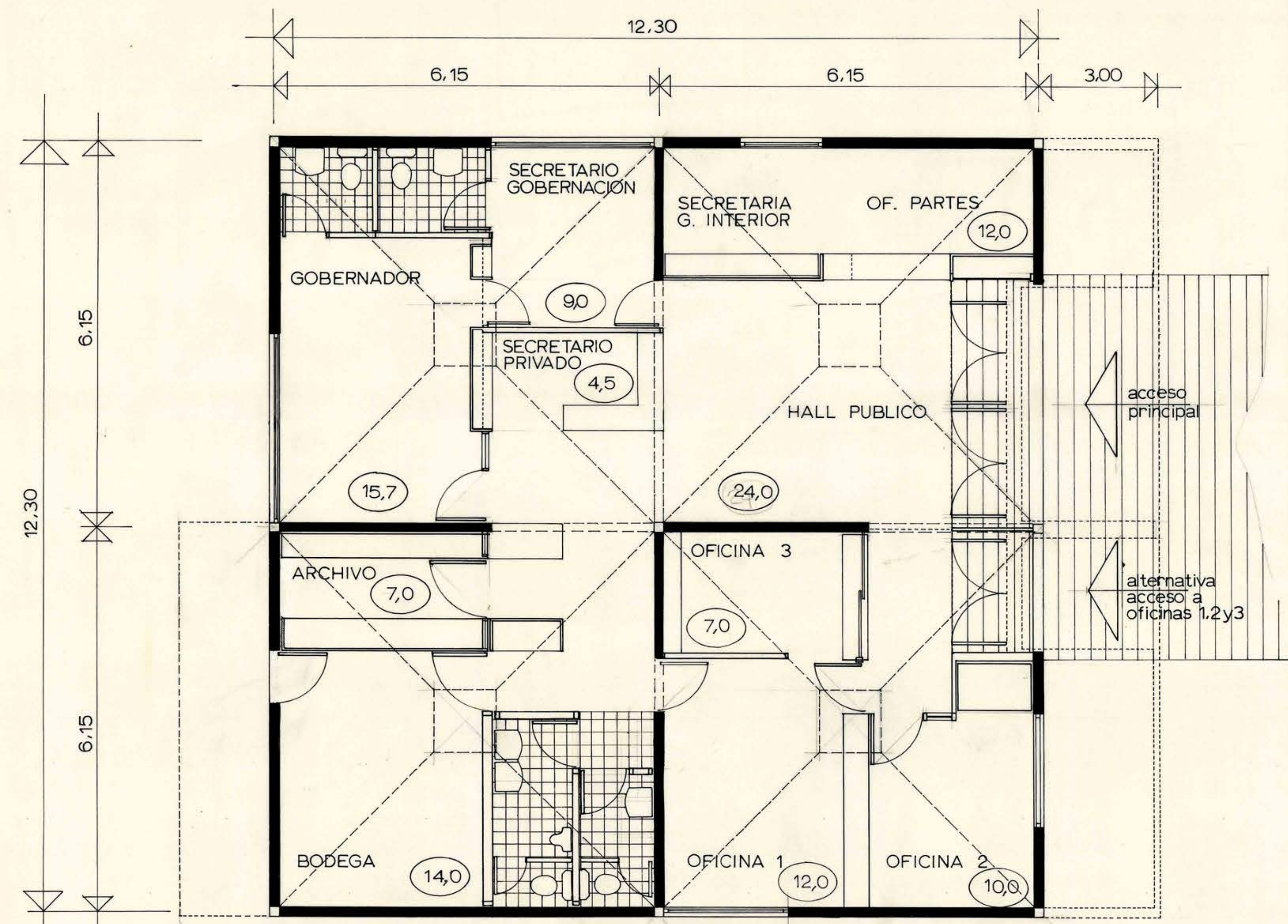
PLANTA
