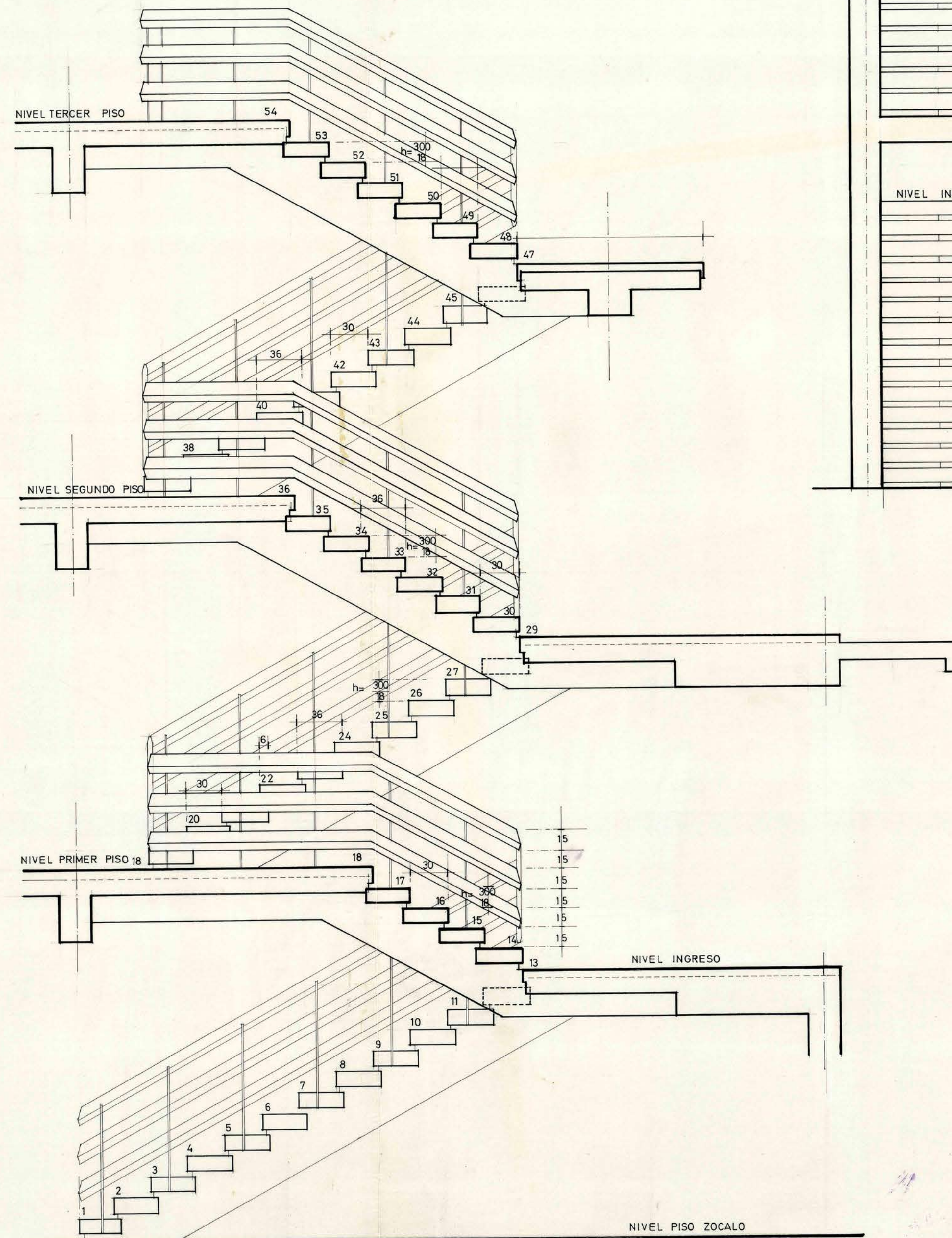
CORTE XX'
