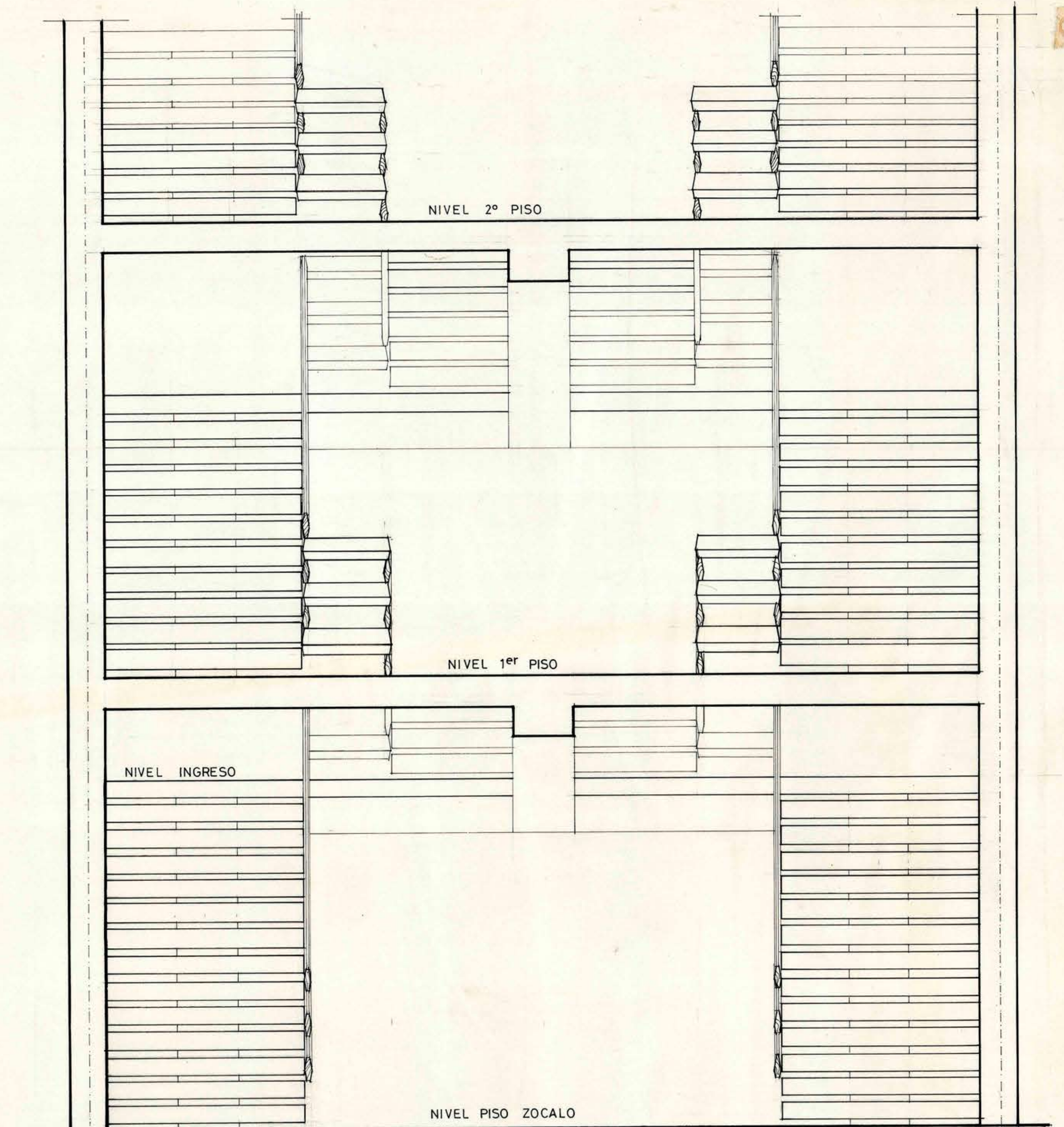
ELEVACION FRONTAL
