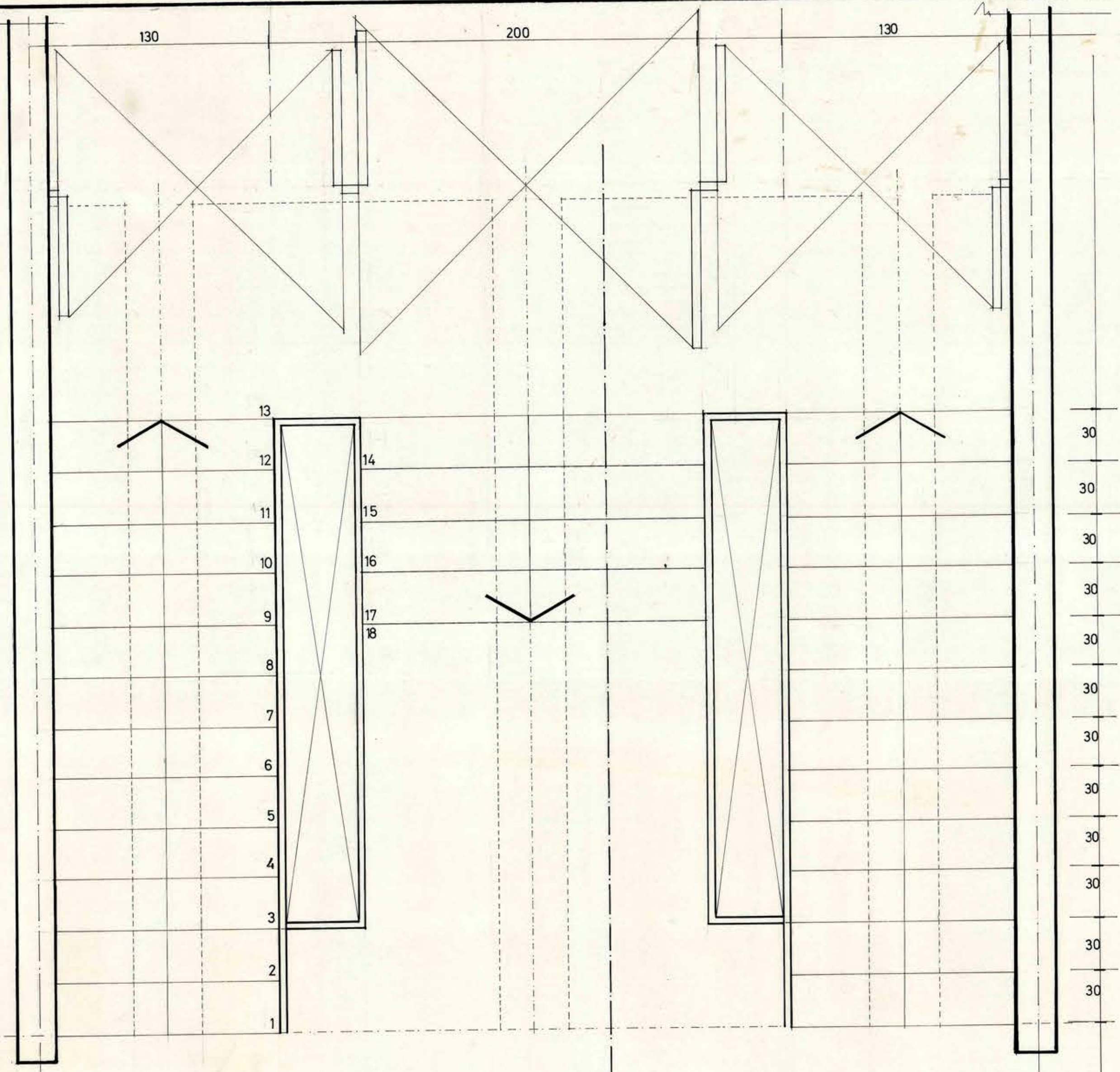
ESCALERA INGRESO PRINCIPAL CORTE XX' TRAMO ZOCALO A PRIMER PISO
