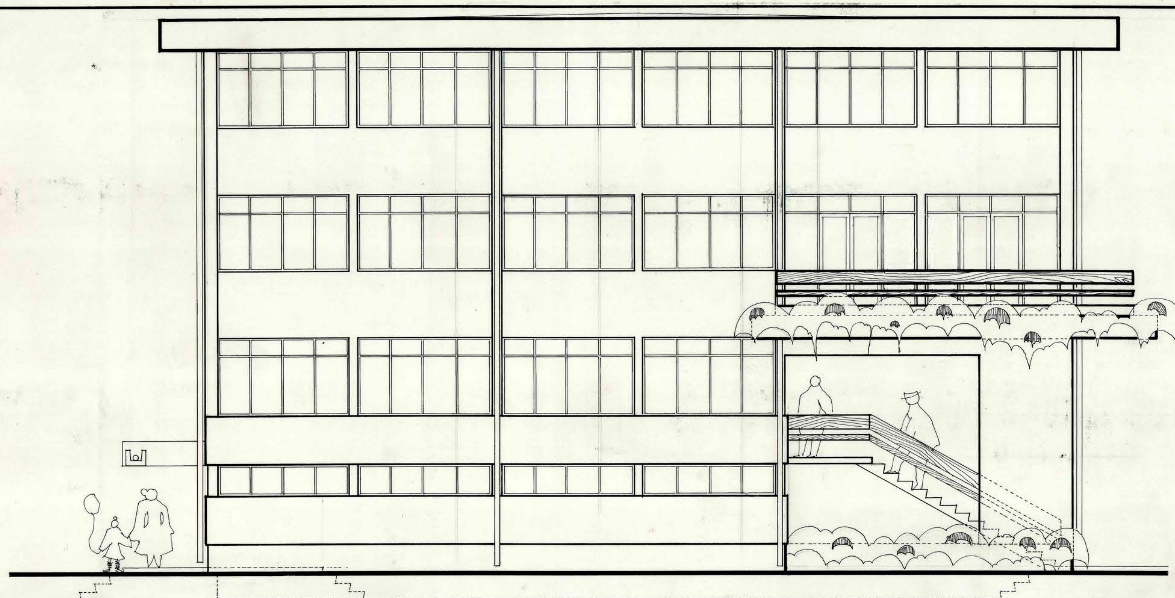
ELEVACION SUR escala 1 / 50
