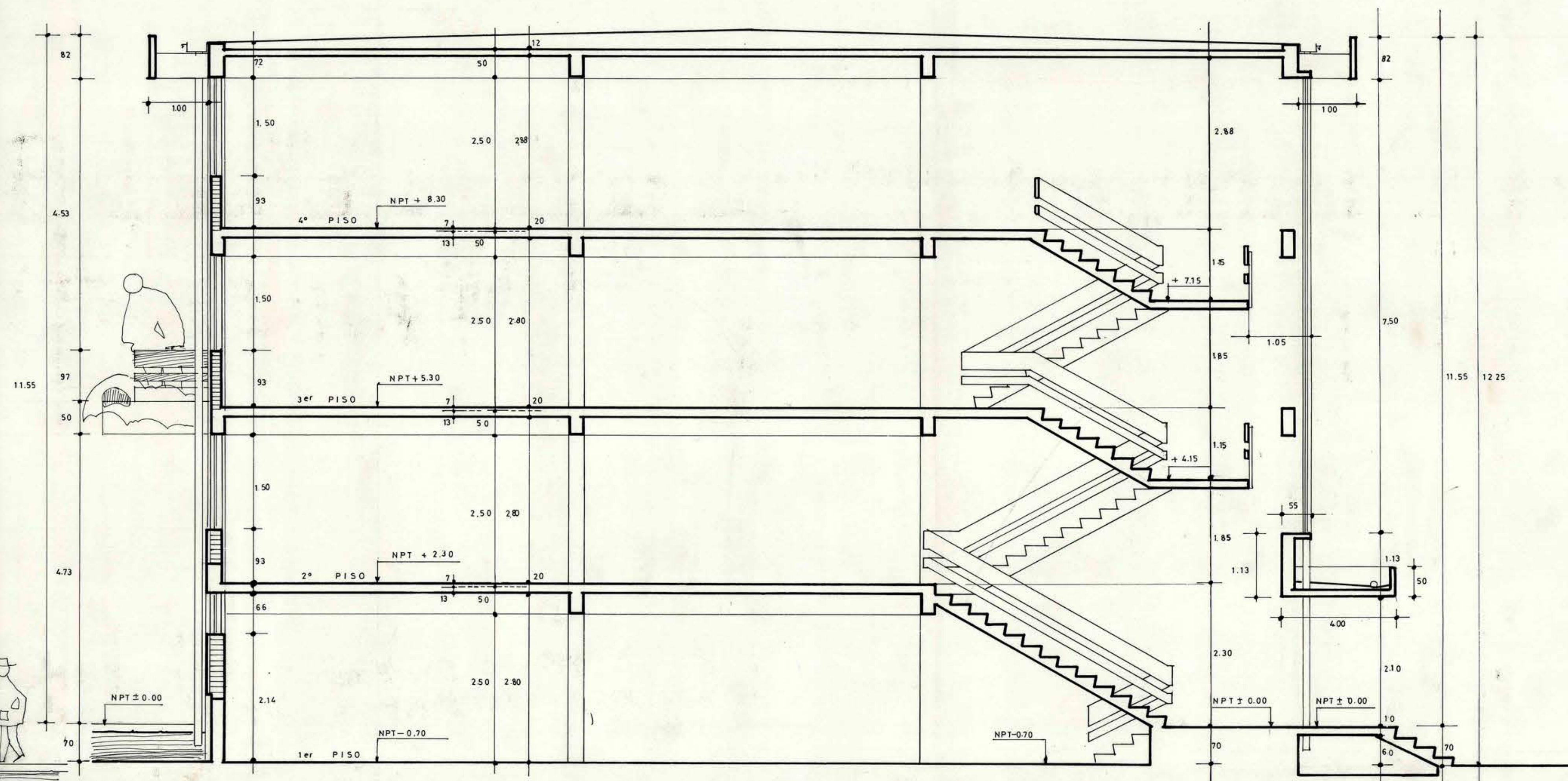
CORTE B-B escala 1 / 50
