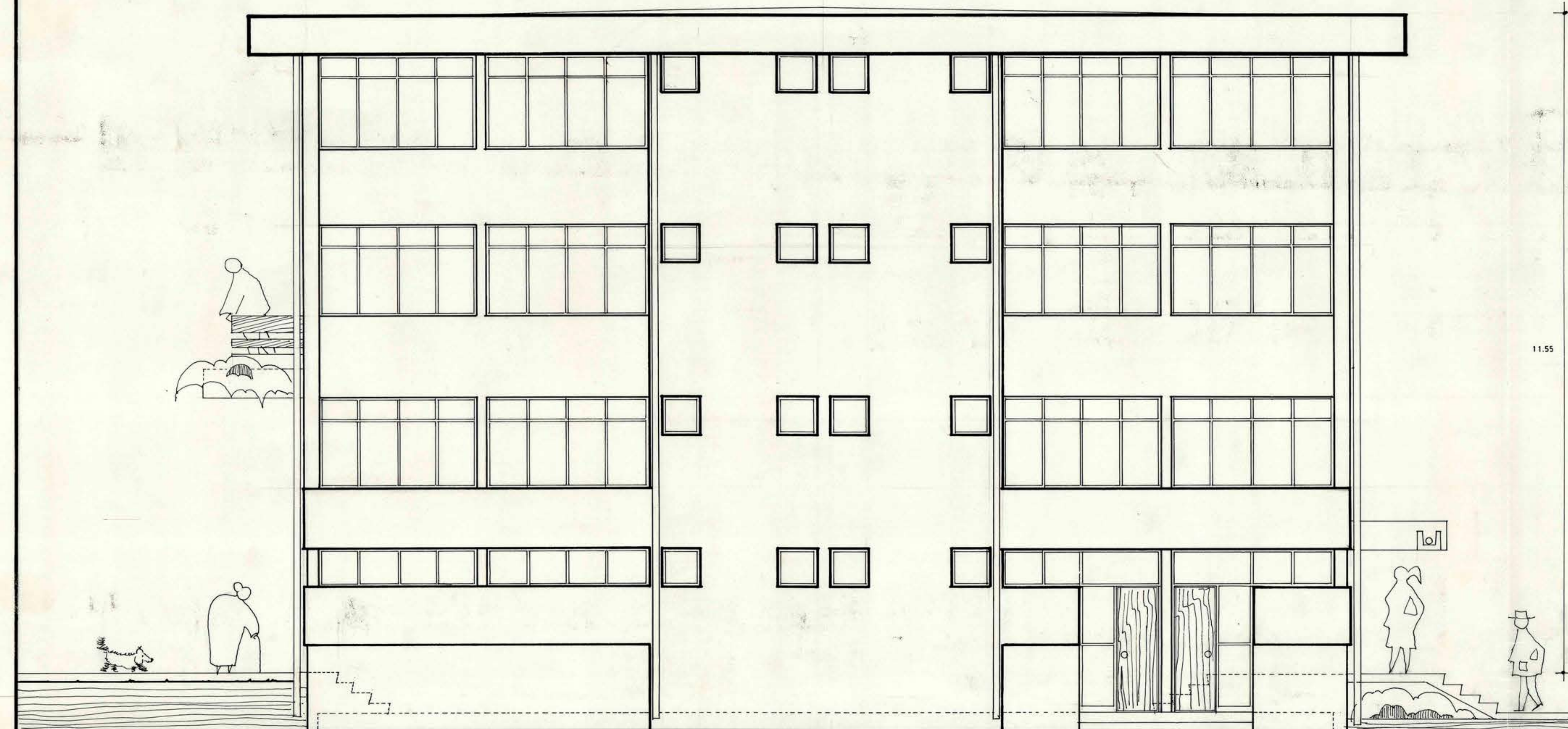
ELEVACION NORTE escala 1 / 50
