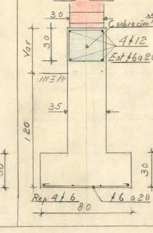
Corte E-E
