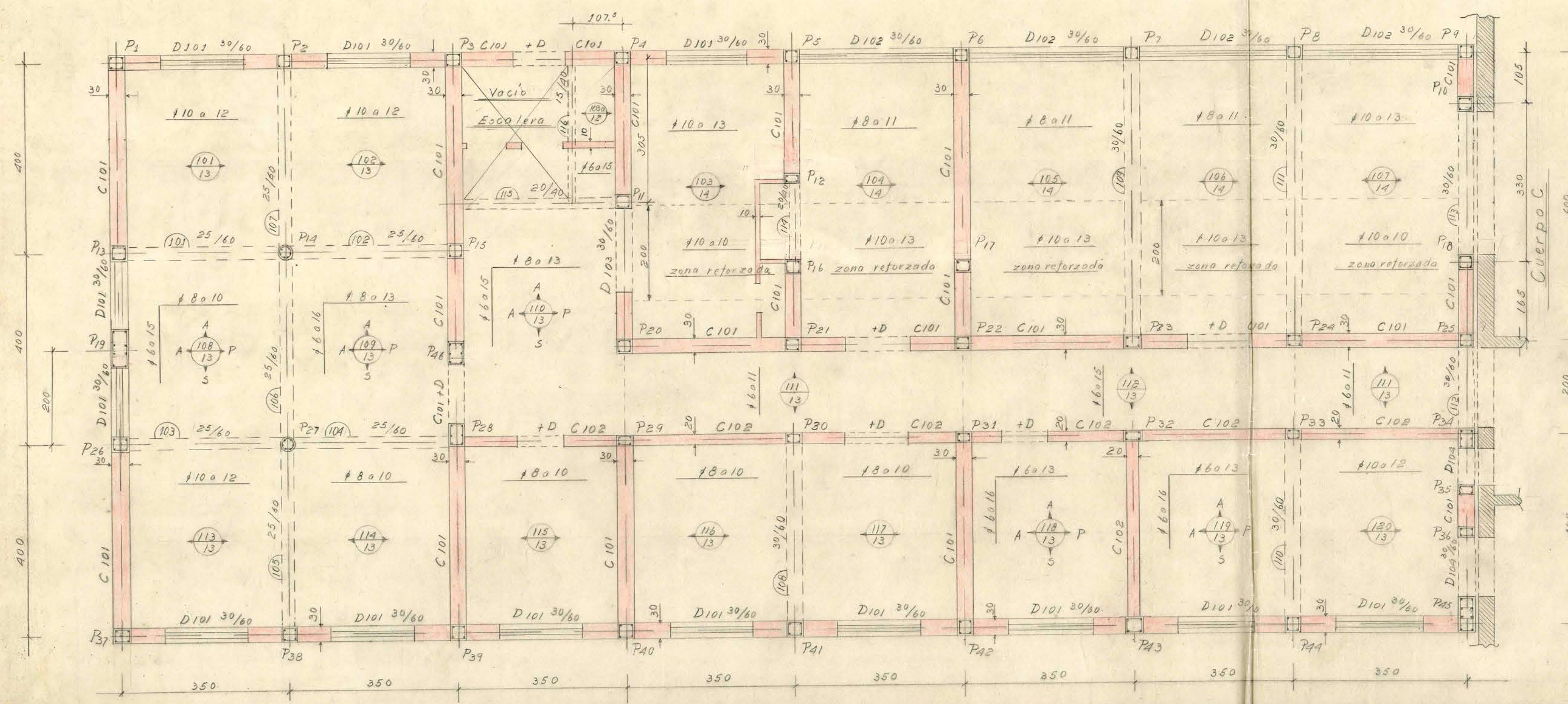
Planta Sobre Primer Piso
