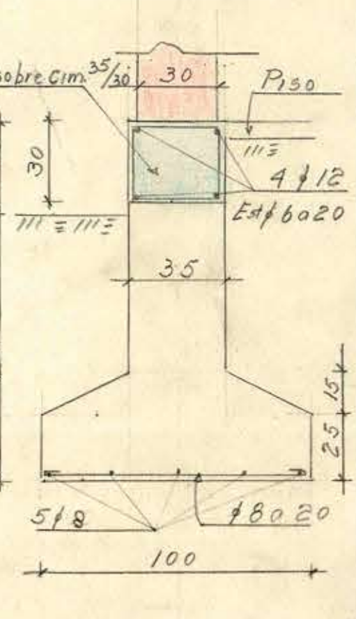
Corte A-A
