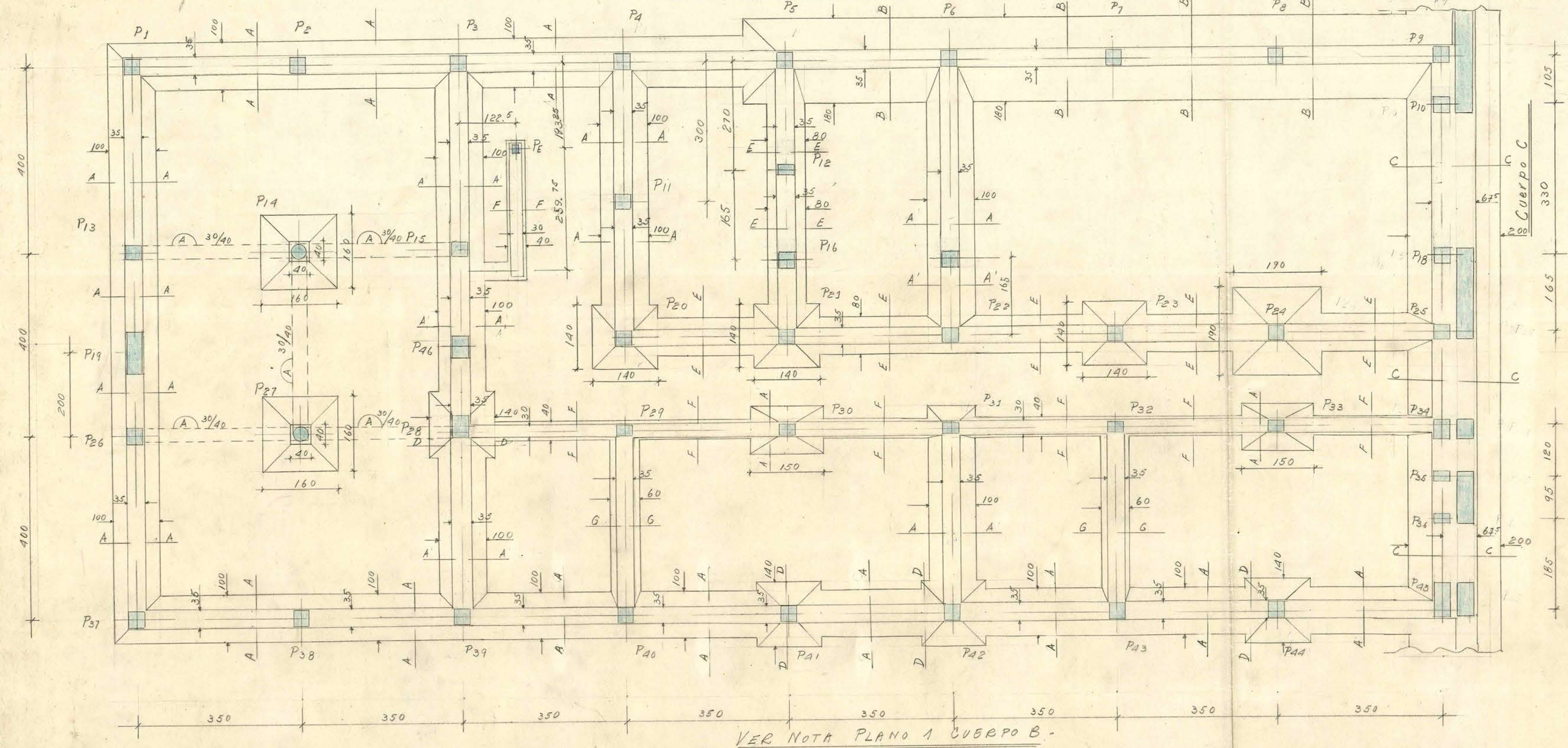
Planta de Fundaciones
