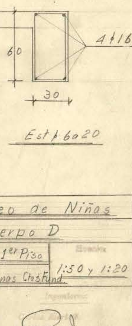
Dintel 102 30/60
