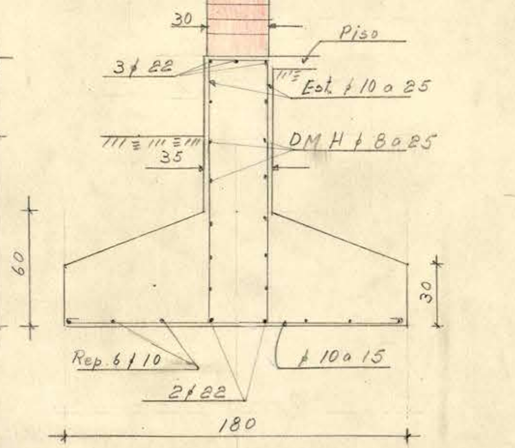
Pilar 20 = 21 = 23
