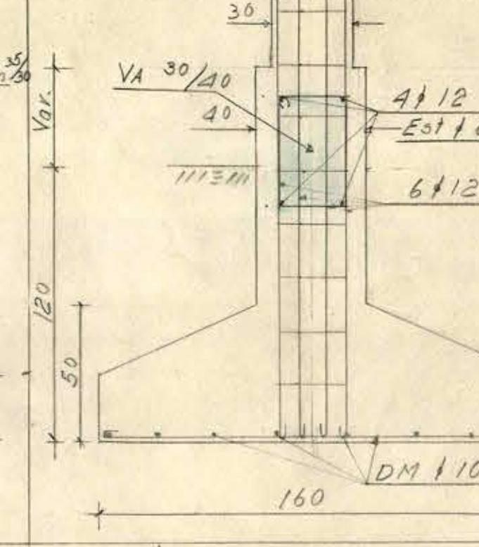
Corte E-E
