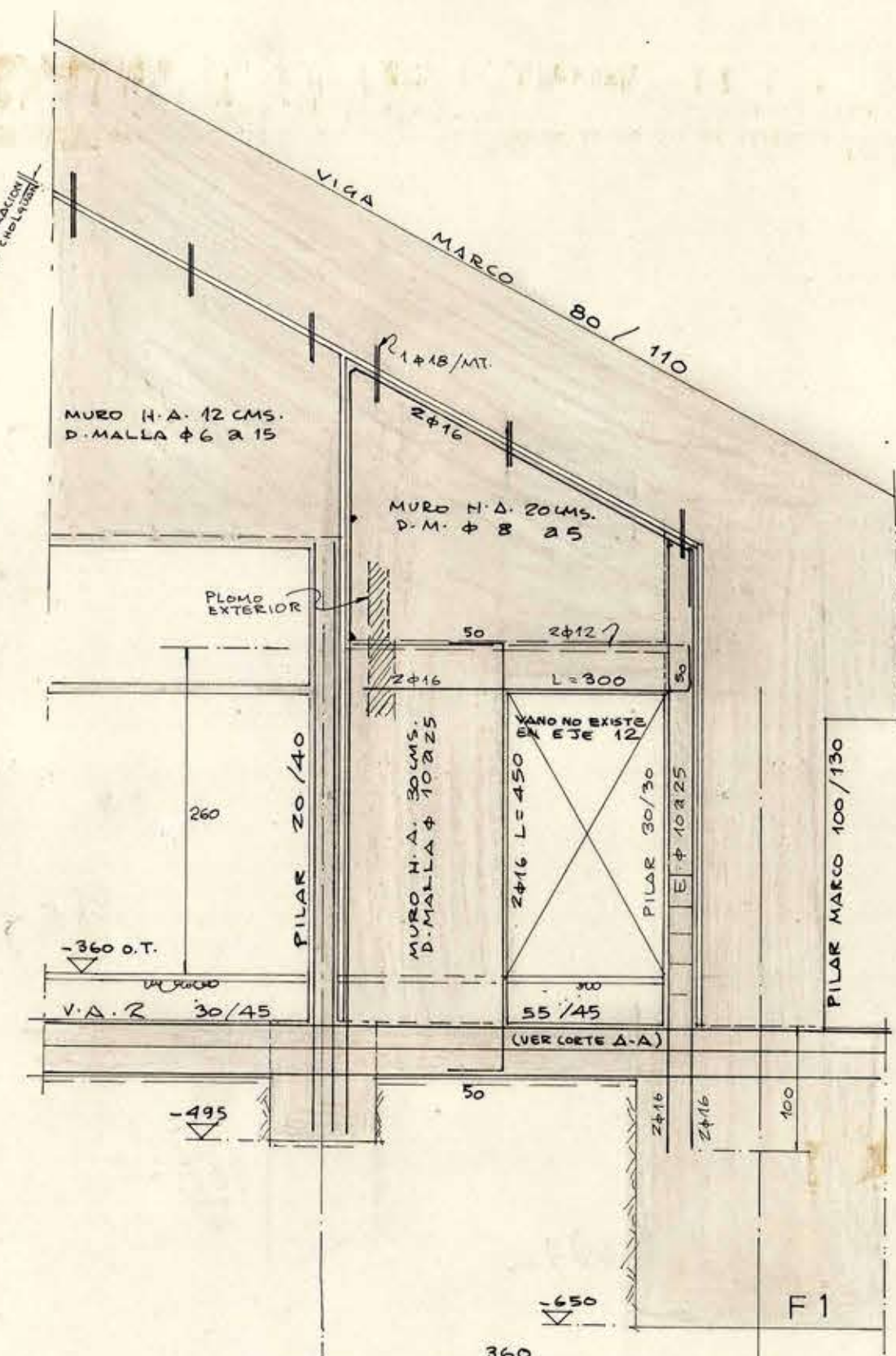
CORTE B - B ESCALA 1 : 50
