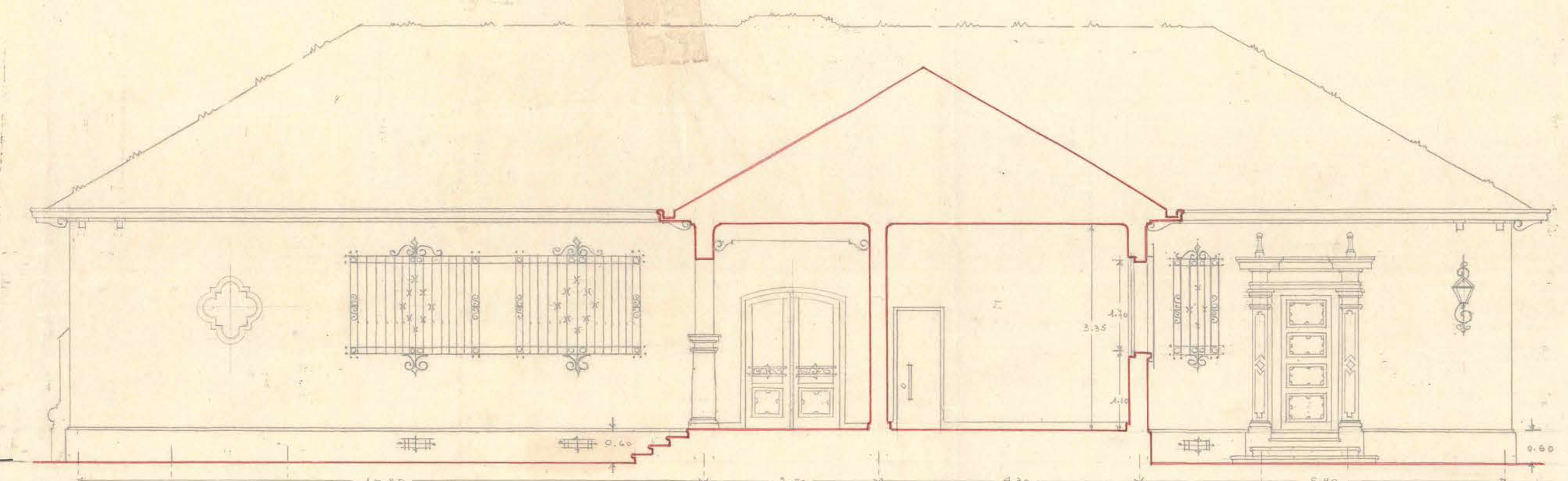
SECCION A-B.
