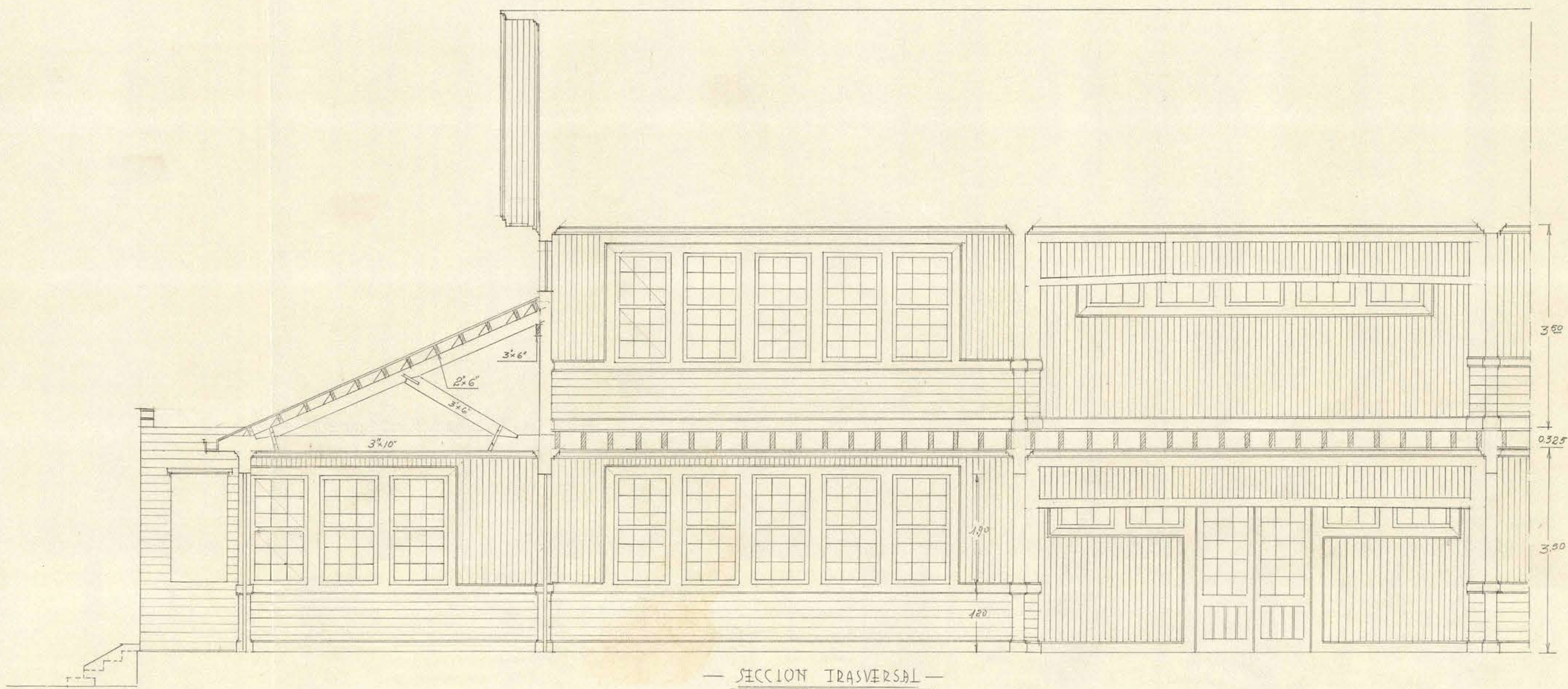
— SECCION TRASVERSAL —
