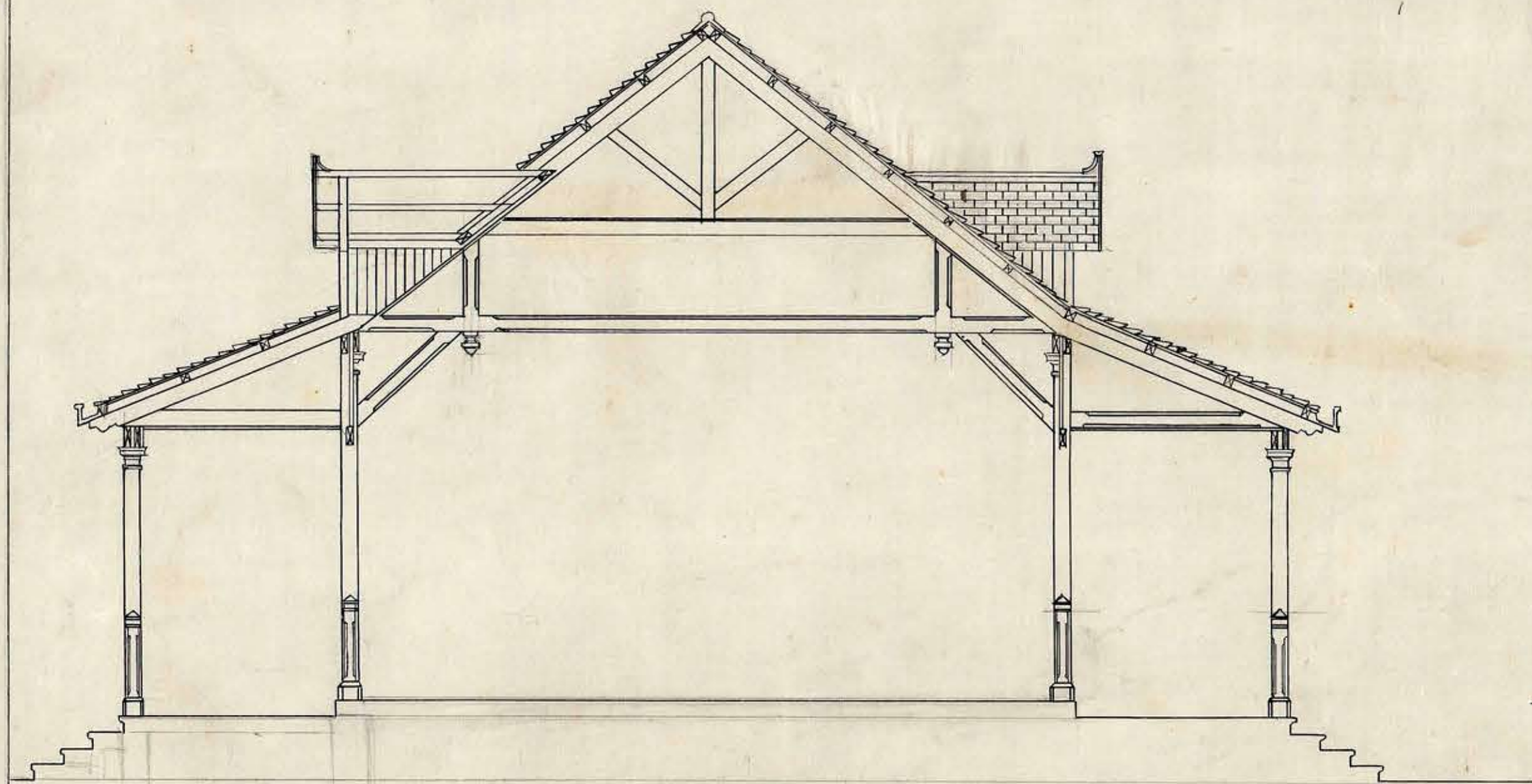
SECCION TRASVERSAL
