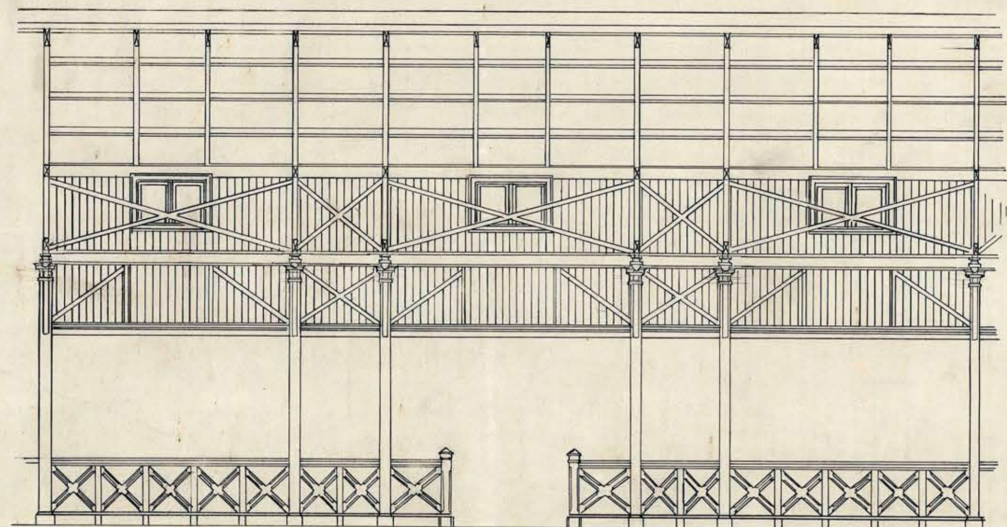
SECCION LONGITUDINAL
