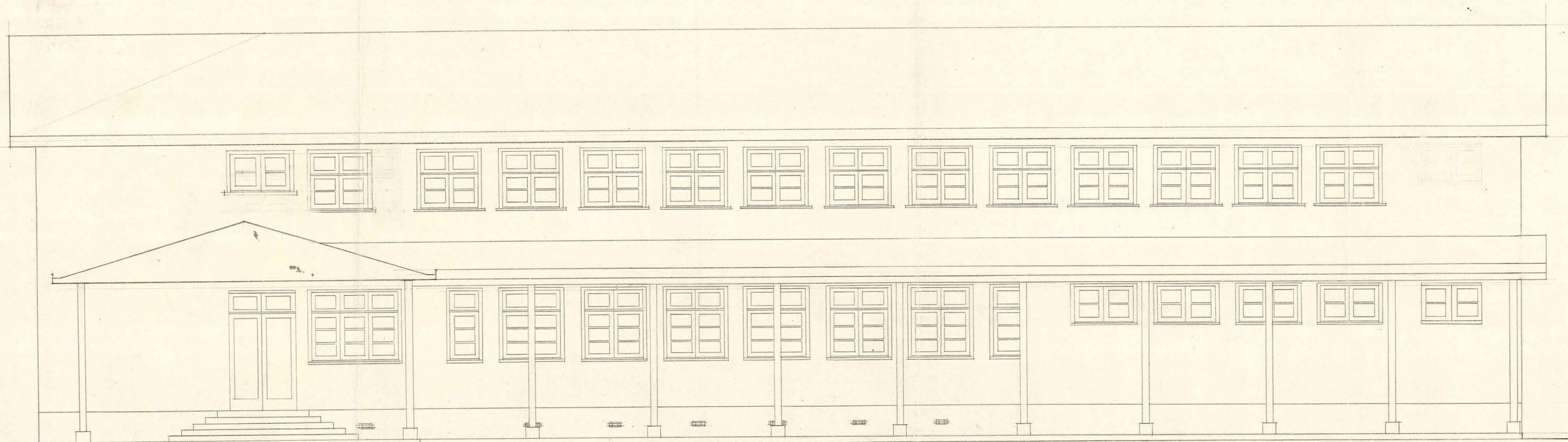
FACHADA ORIENTE
