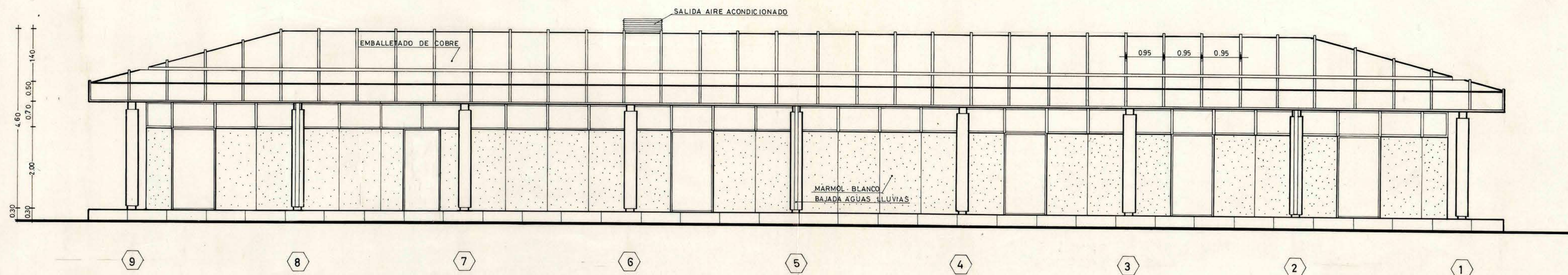
FACHADA SUR
