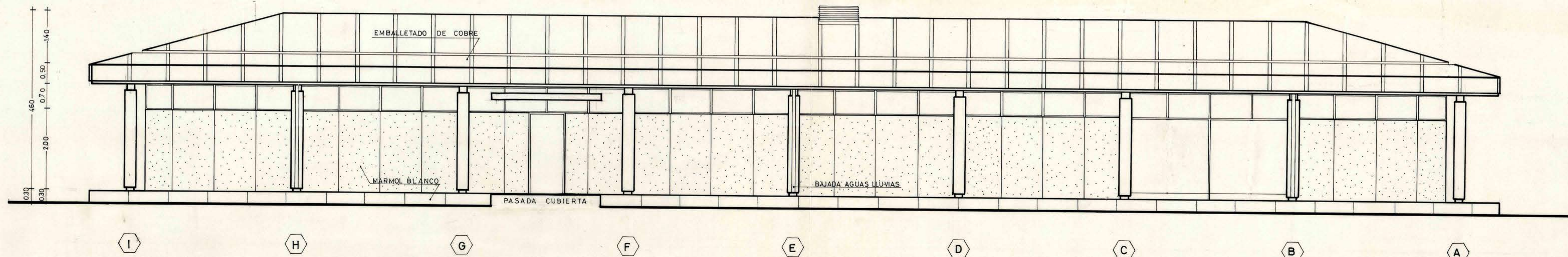
FACHADA ORIENTE
